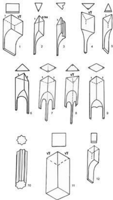
Éléments tridimensionnels des mouquarnas
